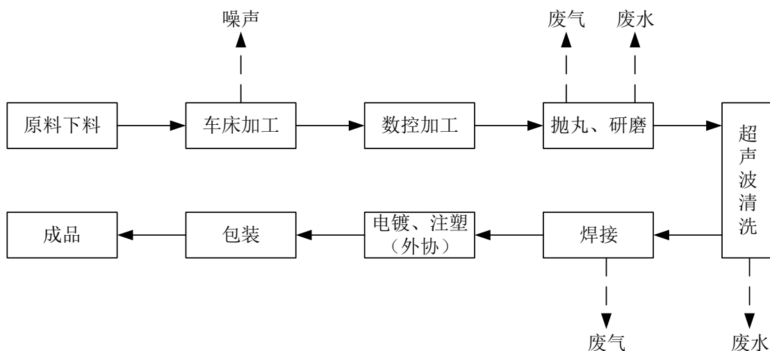
图 1-2 企业生产工艺流程图
